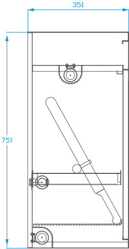
UV BOX E3/40H-NX-C
